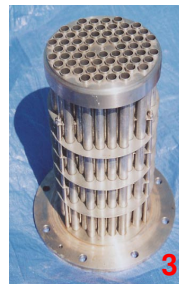
feixe em "U" para trocador com dilatação
