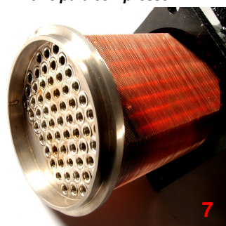
feixe para compressor
