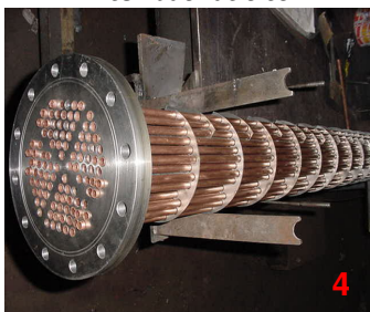
feixe para compressor
