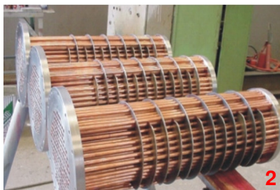
feixe em "U" para trocador com dilatação
