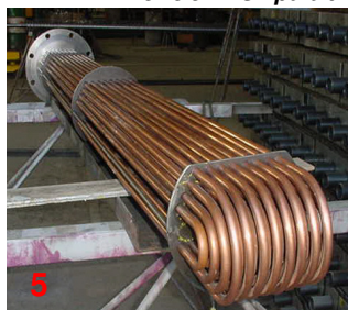
Aquecedor a vapor
